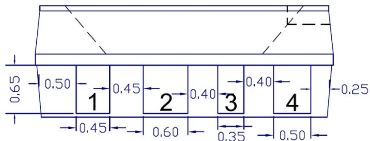
焊盤、焊錫腳示意圖
